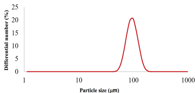
Fig. 2. Particle size distribution of the F1 microspheres.
